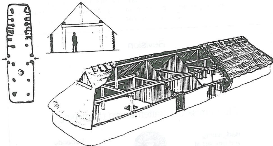
Grundplan, tværsnit og rekonstruktion af jernalderlanghus fra tiden o. Kr.f. (Efter Danmarks Historie bd. 2, 200 f.Kr.-700 e.Kr. Red. Olaf Olsen 1988)
